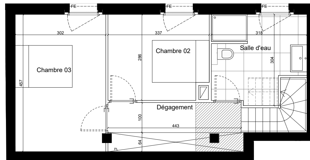
Rez-de-jardin
